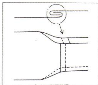
本ハゼ断面図
